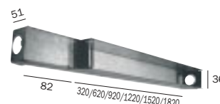
Verschaltung für das Mauerwerk Mounting box Опалубка для кладки
