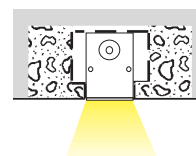
Deckenbündige Einbauleuchte Recessed flush ceiling mounted Встраиваемый блок по потолку
