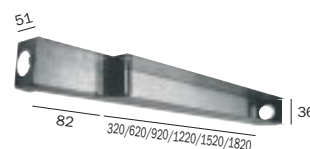
Verschalung für das Mauerwerk Mounting box Опалубка для кладки
